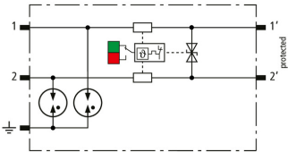
Schéma vnitřního zapojení BCO MOD ML2 BD 48
