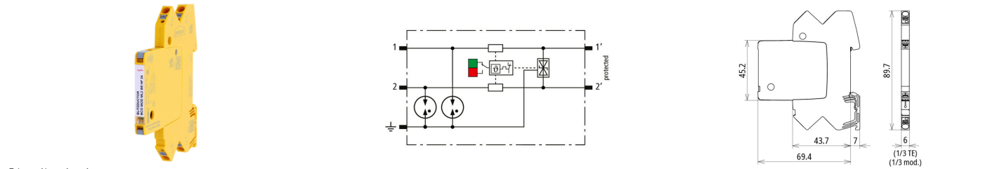
Zobrazení je nezávazné Schéma zapojení BCO ML2 BE HF 24 Rozměry BCO ML2 BE HF 24
