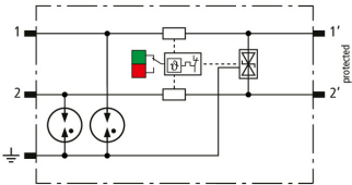
Schéma vnitřního zapojení BCO ML2 BE HF 5
