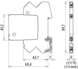
Rozměry BCO ML2 BE HF 5
