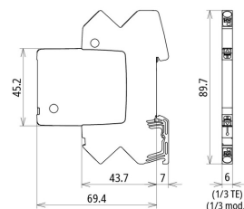
Rozměry BCO ML2 BD 48
