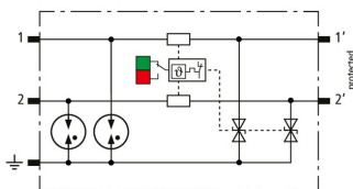
Schéma vnitřního zapojení BCO ML2 BE 180
