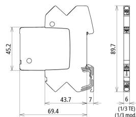
Rozměry BCO ML2 BE 24
