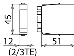
Rozměry BXT ML2 BD DL S 15
