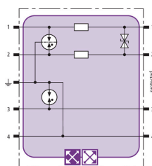
Schéma vnitřního zapojení BXT ML2 BD DL S 15
