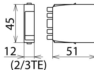
Rozměry BXT ML2 B 180
