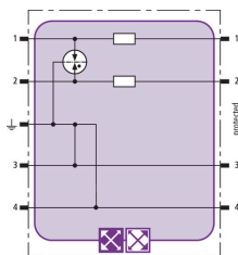
Schéma vnitřního zapojení BXT ML2 B 180
