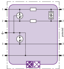
Schéma vnitřního zapojení BXT ML2 BD HFS 5
