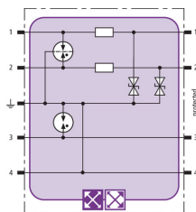
Schéma vnitřního zapojení BXT ML2 BE S 24
