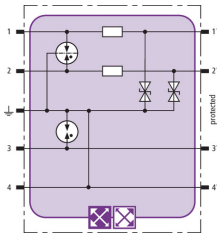
Schéma vnitřního zapojení BXT ML2 BE S 5
