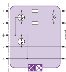
Schéma vnitřního zapojení BXT ML2 BD S 24
