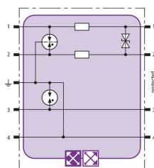
Schéma vnitřního zapojení BXT ML2 BD S 12
