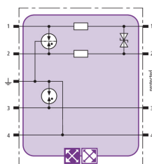
Schéma vnitřního zapojení BXT ML2 BD S 5
