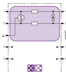
Schéma vnitřního zapojení BXT ML2 BD 180
