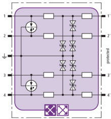
Schéma vnitřního zapojení BXT ML4 BE C 24
