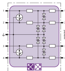
Schéma vnitřního zapojení BXT ML4 BE C 12
