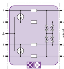
Schéma vnitřního zapojení BXT ML4 BC 24
