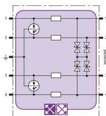
Schéma vnitřního zapojení BXT ML4 BC 5
