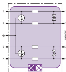
Schéma vnitřního zapojení BXT ML4 BD 180
