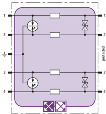
Schéma vnitřního zapojení BXT ML4 BD 24
