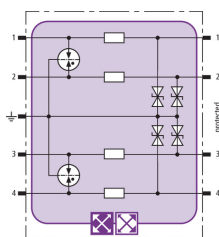
Schéma vnitřního zapojení BXT ML4 BE 180
