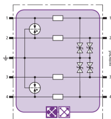
Schéma vnitřního zapojení BXT ML4 BE 36
