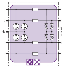
Schéma vnitřního zapojení BXT ML4 BC EX 24
