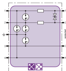
Schéma vnitřního zapojení BXT ML2 BD S EX 24
