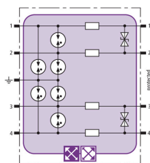
Schéma vnitřního zapojení BXT ML4 BD EX 24
