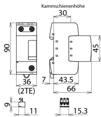
Rozměry DSE M 1 242 FM
