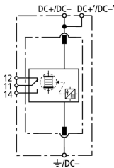
Schéma vnitřního zapojení DSE M 1 242 FM
