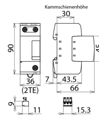
Rozměry DSE M 1 220 FM
