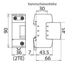
Rozměry DSE M 1 60
