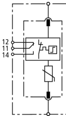
Schéma vnitřního zapojení DG S 385 FM
