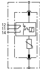
Schéma vnitřního zapojení DG S 320 FM
