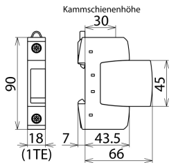
Rozměry DG S 48
