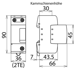
Rozměry DB M 1 150
