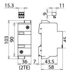
Rozměry DG 1000 FM
