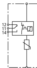
Schéma vnitřního zapojení DG 1000 FM
