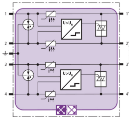
Schéma vnitřního zapojení BXTU ML4 BD 0-180
