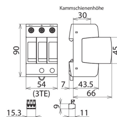
Rozměry DG M YPV SCI 1000 FM
