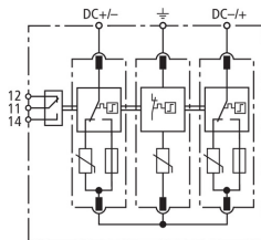
Schéma vnitřního zapojení DG M YPV SCI 1000 FM
