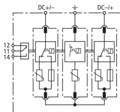
Schéma vnitřního zapojení DG M YPV SCI 150 FM
