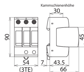
Rozměry DG M YPV SCI 1200
