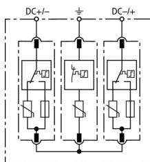
Schéma vnitřního zapojení DG M YPV SCI 1200
