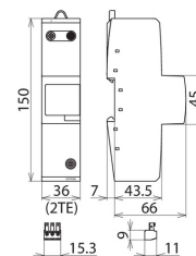
Rozměry DVCI 1 255 FM
