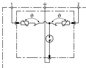
Schéma vnitřního zapojení DR M 2P 255 SN1802
