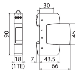
Rozměry DR M 2P 255 SN1802
