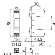
Rozměry DR M 2P 255 FM
