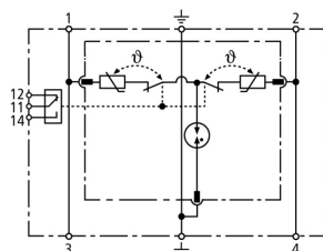
Schéma vnitřního zapojení DR M 2P 255 FM
