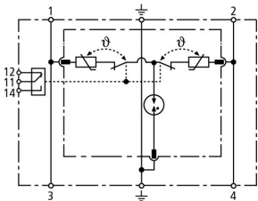
Schéma vnitřního zapojení DR M 2P 75 FM
