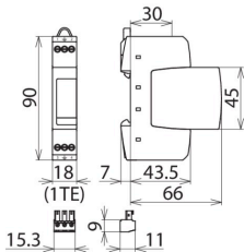
Rozměry DR M 2P 75 FM
