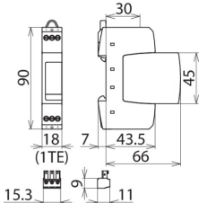
Rozměry DR M 2P 60 FM
