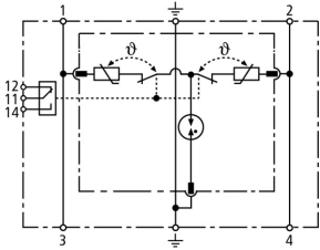
Schéma vnitřního zapojení DR M 2P 60 FM
