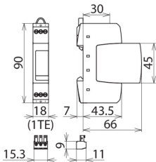
Rozměry DR M 2P 30 FM
