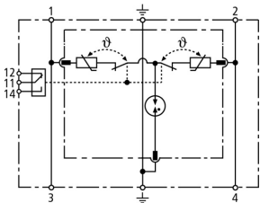
Schéma vnitřního zapojení DR M 2P 30 FM
