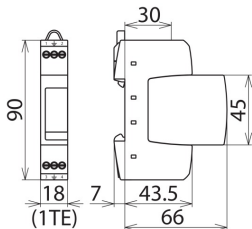
Rozměry DR M 2P 255
