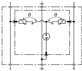
Schéma vnitřního zapojení DR M 2P 255
