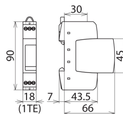
Rozměry DR M 2P 150
