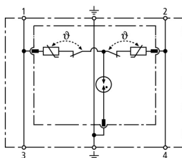
Schéma vnitřního zapojení DR M 2P 150
