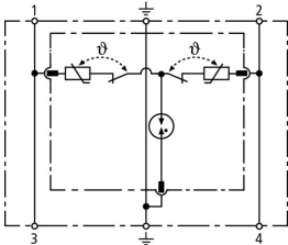
Schéma vnitřního zapojení DR M 2P 75
