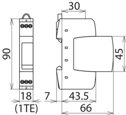
Rozměry DR M 2P 75
