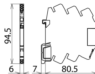
Rozměry DCO SD2 E 48
