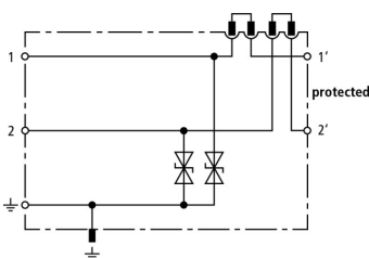
Schéma vnitřního zapojení DCO SD2 E 24
