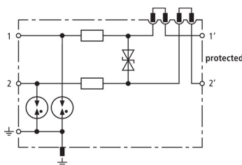
Schéma vnitřního zapojení DCO SD2 MD 48
